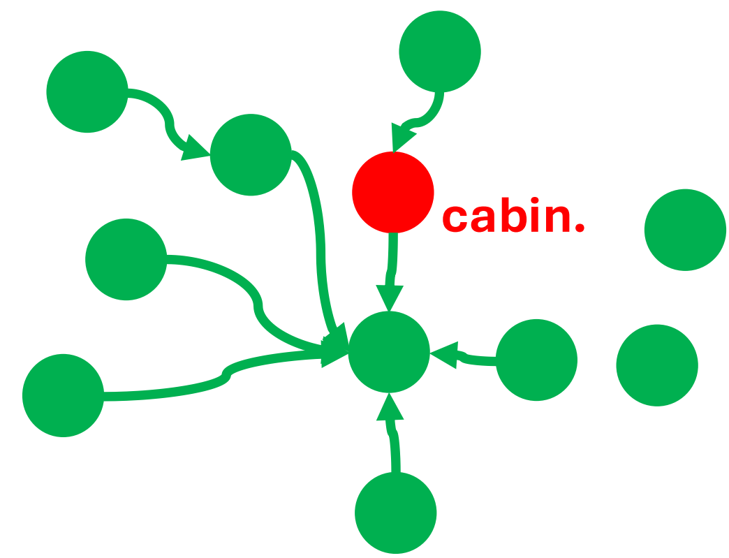
NoPA (Ours)
